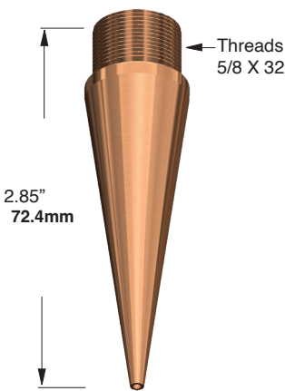
Nozzle 603-271-003 1.5mm 603-271-005
