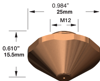
Nozzle EAA
